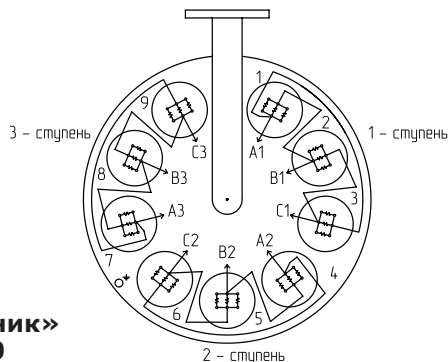
Рис.2 Расположение выводов и схема подключения электроводонагревателя.
