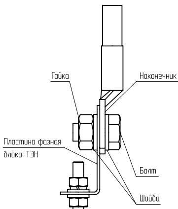
Рис.3 Присоединение проводов к выводам блок-ТЭН
